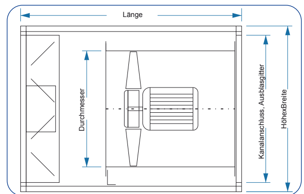
Ventilatorbox, aussen
