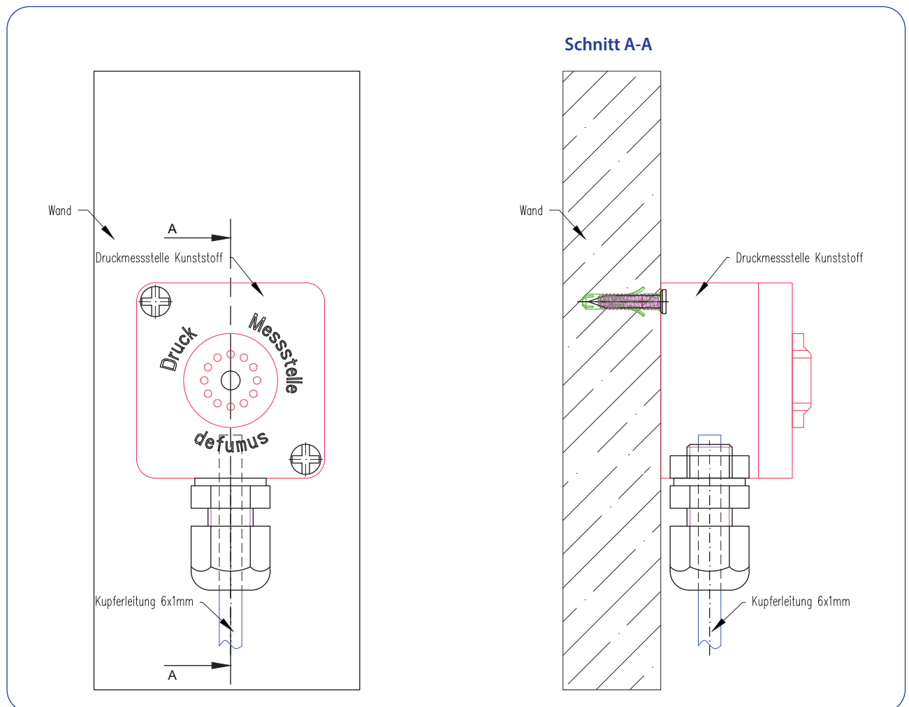
Druckmessstelle, Standardausführung
