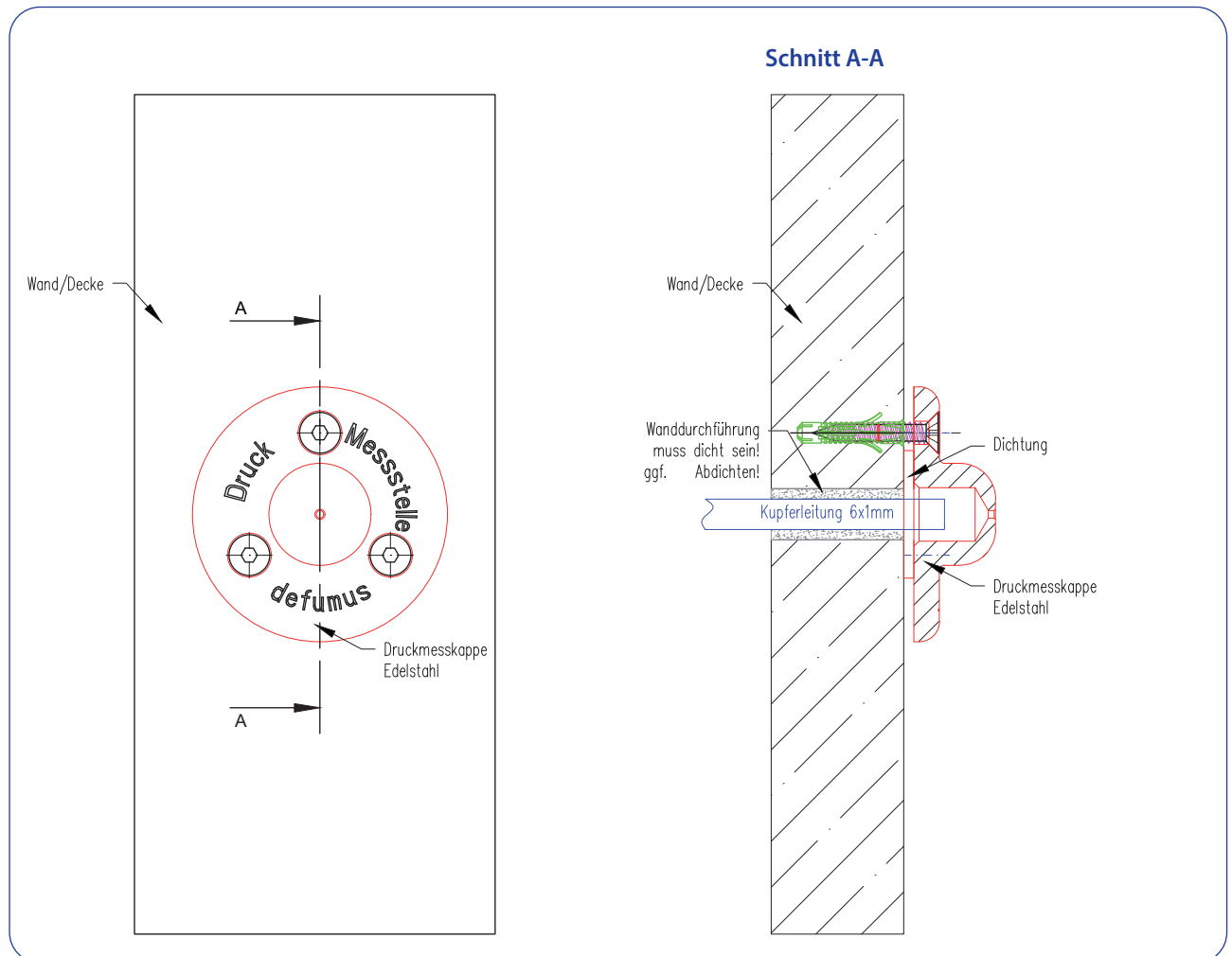
Druckmessstelle, alternative Ausführung
