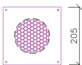
Abdeckgitter 205x205mm mit Montagerahmen 15mm
