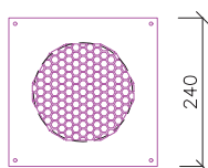
Abdeckgitter 240x240mm mit Montagerahmen 15mm
