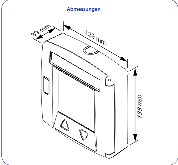
Handbedienstelle RT45
